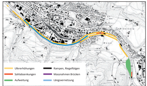
Massnahmen-Übersicht Wasserbauplan Iflis Langnau Mitte-Ost.
